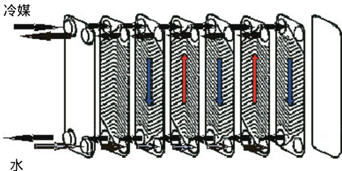
图.9 平板式热交换器的结构示意图
